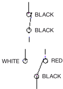
LEM5CNSC SPDT CONTACT
