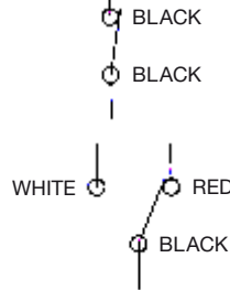
LEM6LNCS SPDT CONTACT
